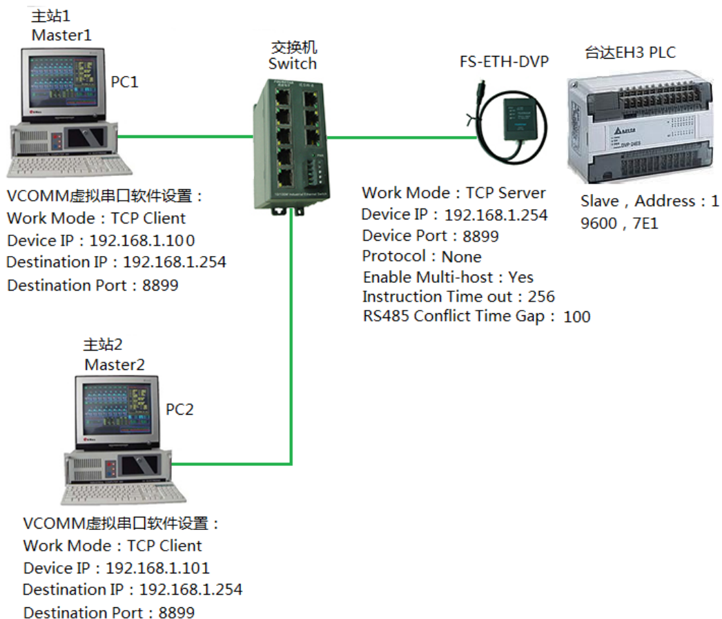
图 1-1 组态王与台达 EH3 PLC 多主站通讯连接拓扑
