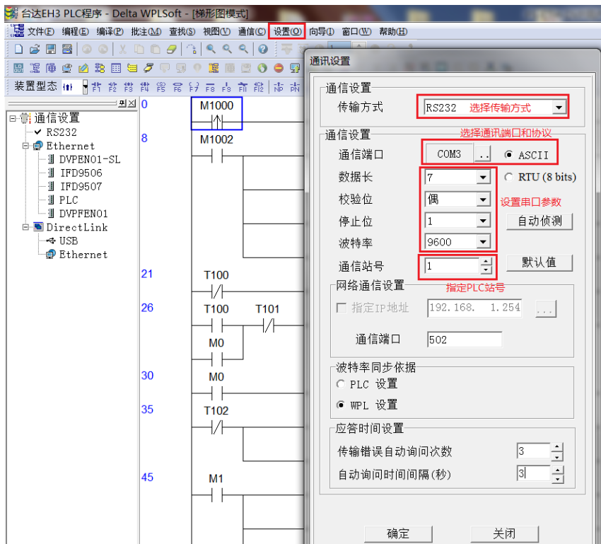
图 5.1-3 台达 PLC 编程软件中的设置
