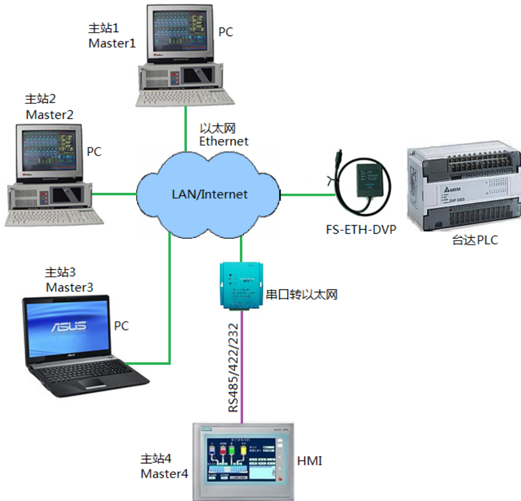
图 1-2 采用 FS-ETH-DVP 的多主站通讯网络拓扑
