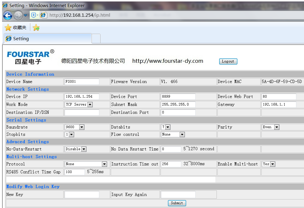
图 1-2 FS-ETH-DVP 参数设置截图
