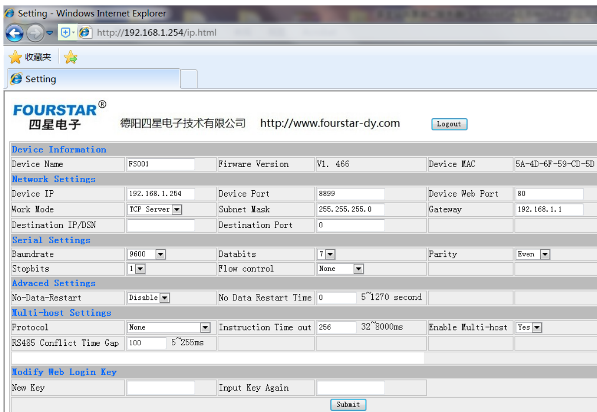
图5.2-1 FS-ETH-DVP作多主站共享串口服务器时的设置
