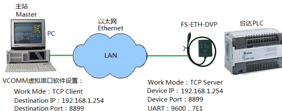
图5.1-1 计算机与台达PLC通过以太网通讯
