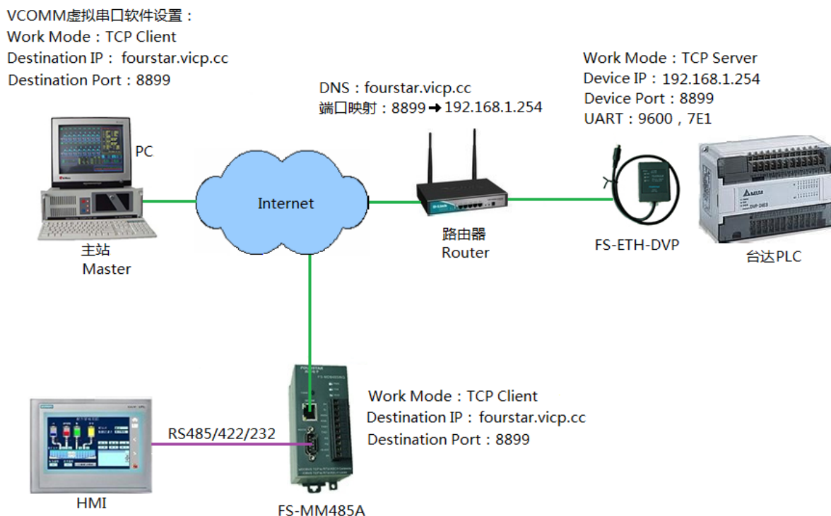
图5.3-1 FS-ETH-DVP在互联网上的通讯网络拓扑
