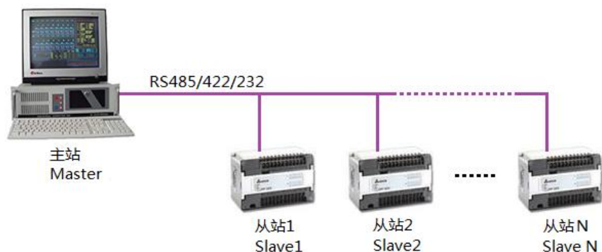
图 1-1 典型的单个主站 RS485 通讯网络拓扑
